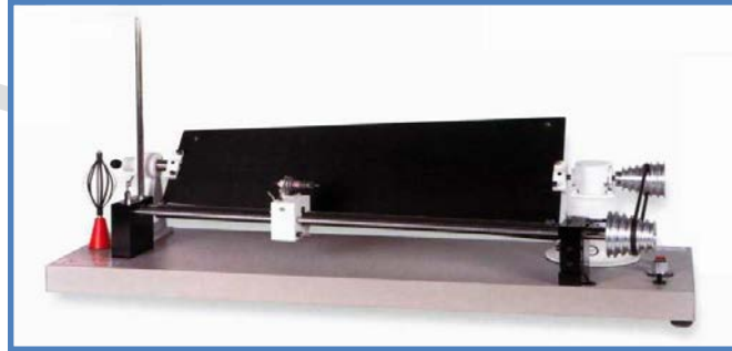
Resim 1.4: Subjektif düzgünsüzlük test cihazı
